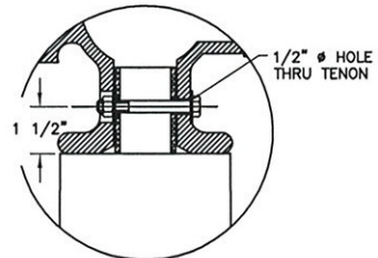
TENON DETAIL SCALE: 4:1
