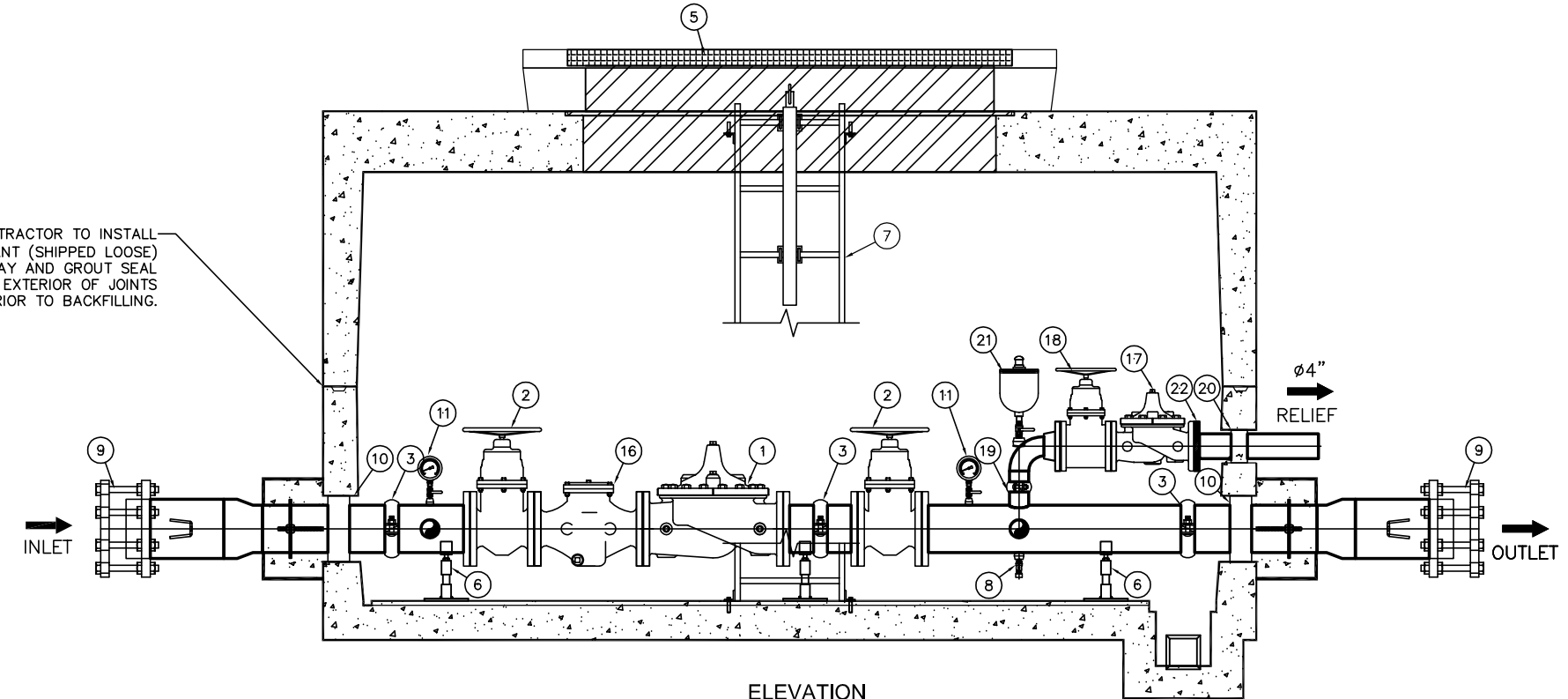
ELEVATION
