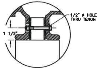
TENON DETAIL SCALE: 4:1
